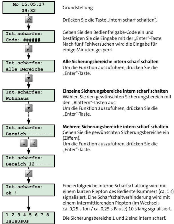
Intern scharf schalten
