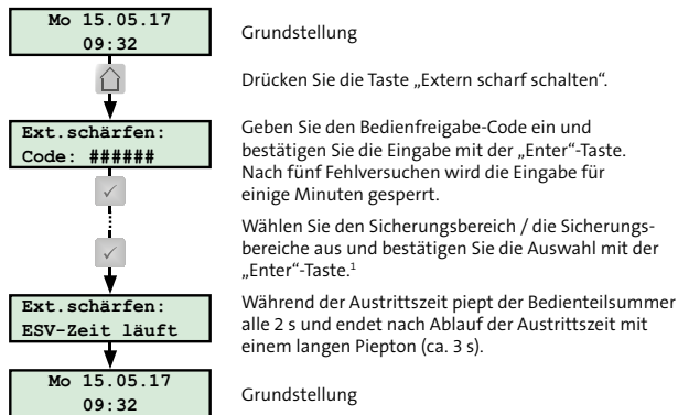
Extern scharf schalten mit Schleusenfunktion
